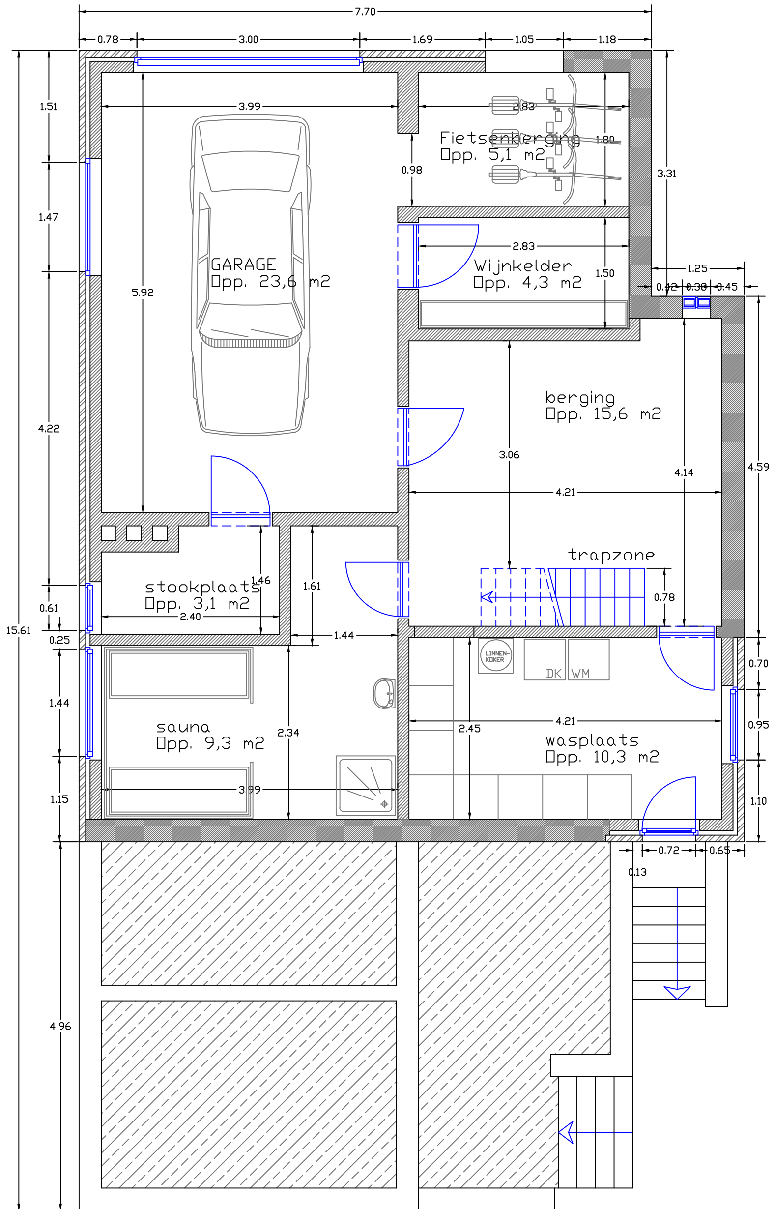
GRONDPLAN KELDER
