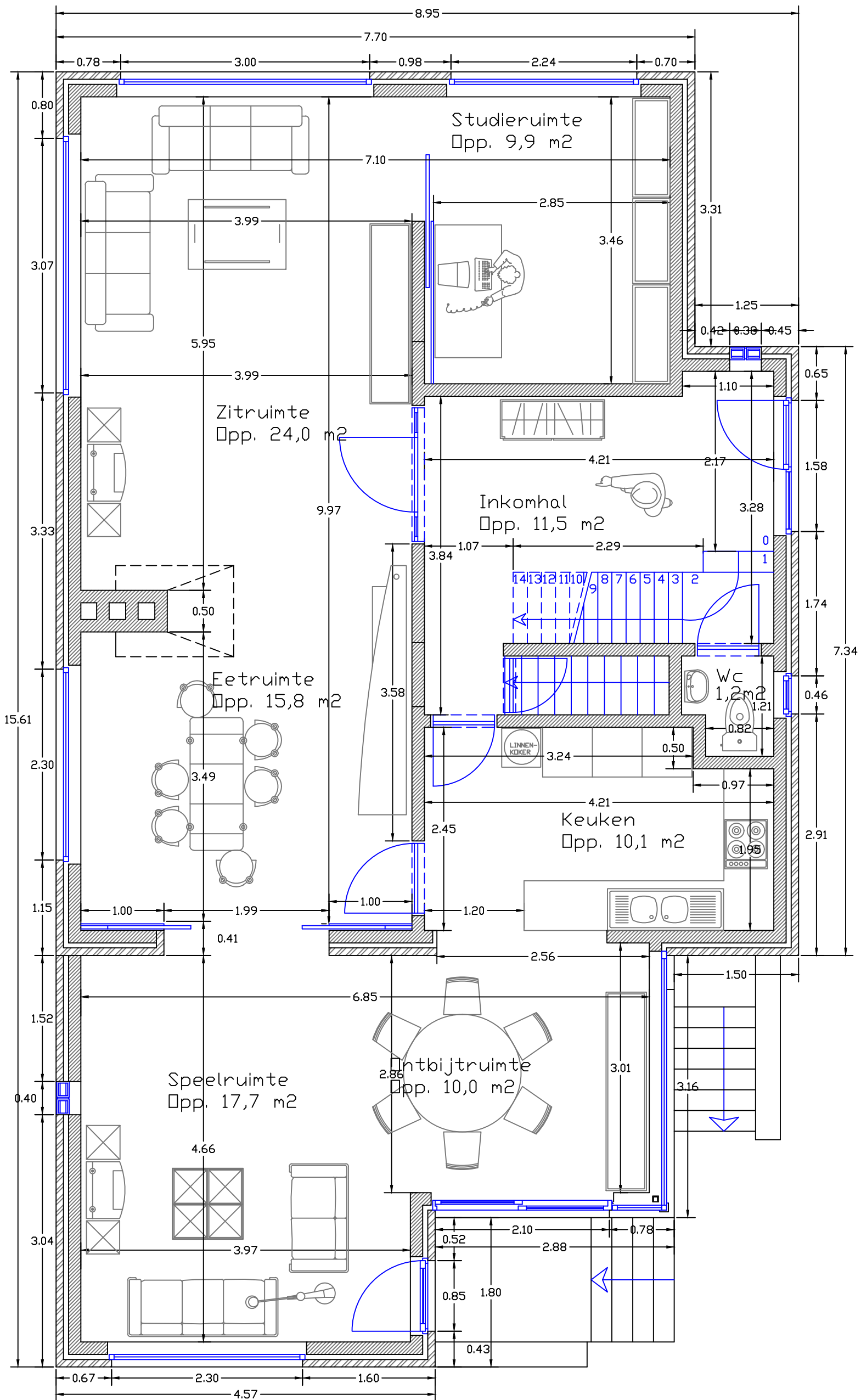
GRONDPLAN GELIJKVLOERS
