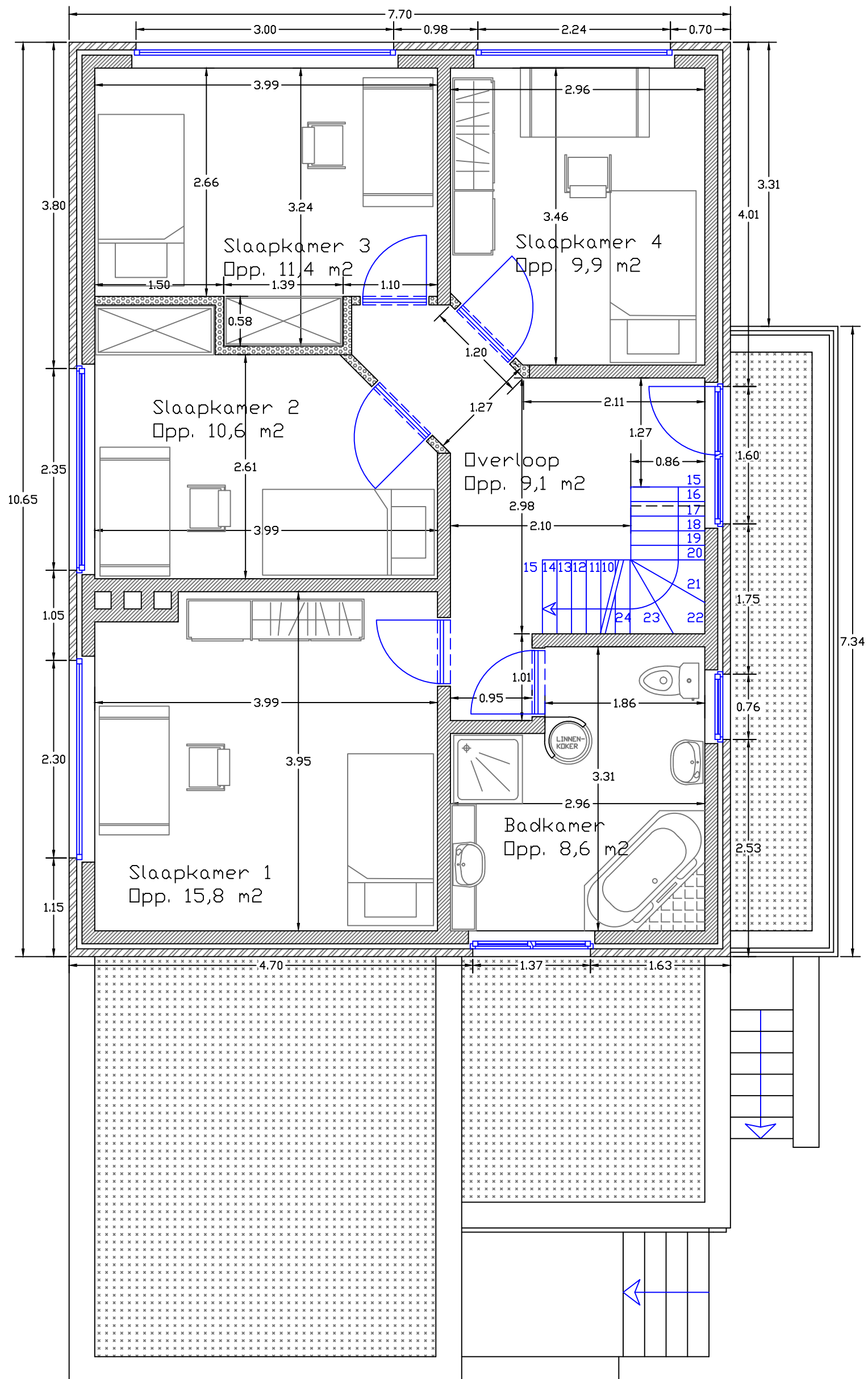
GRONDPLAN EERSTE VERDIEPING
